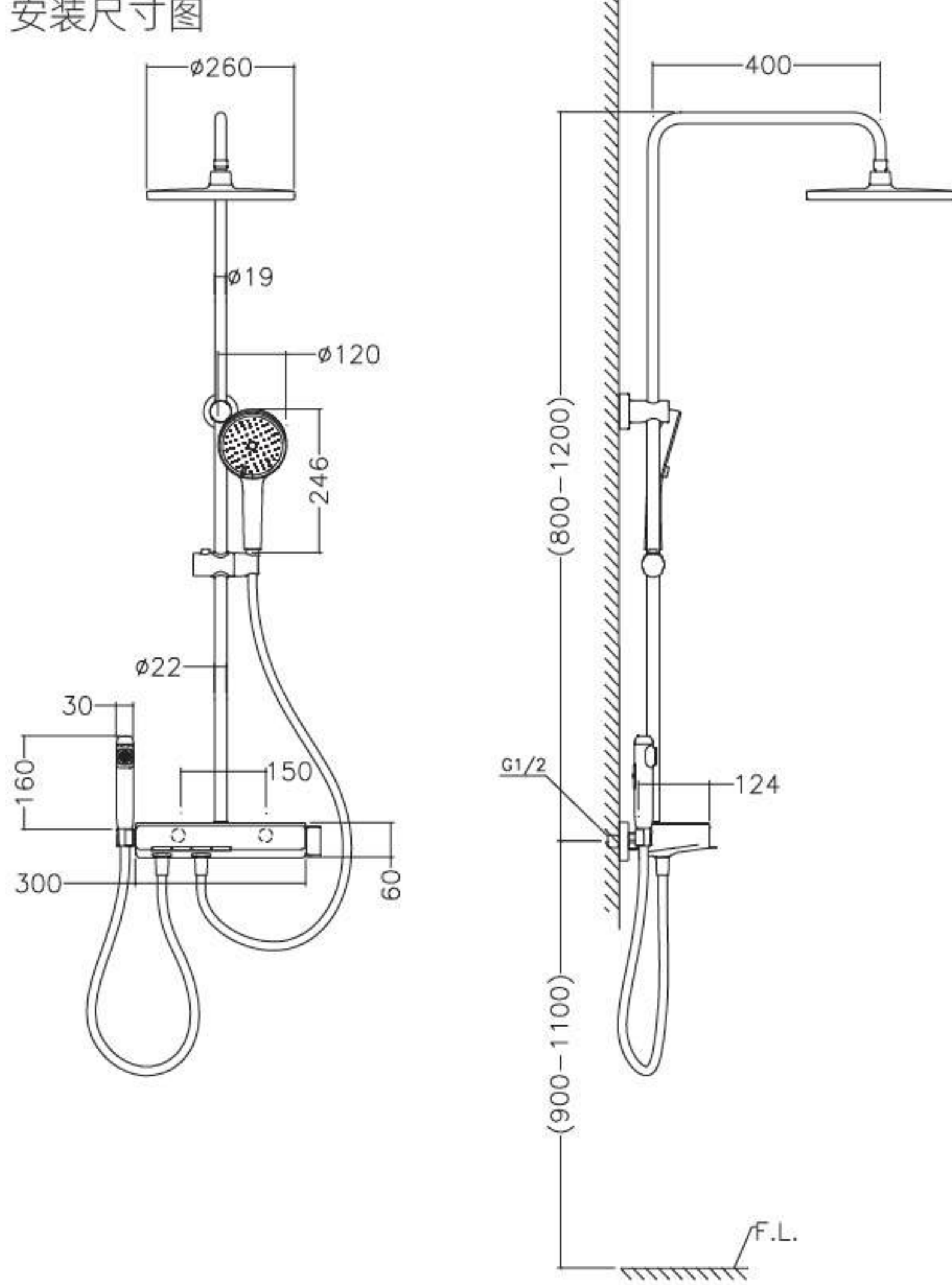
安装尺寸图
