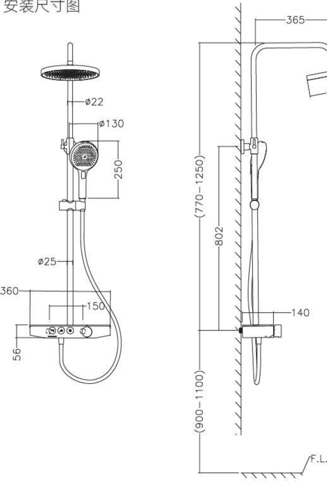
安装尺寸图
