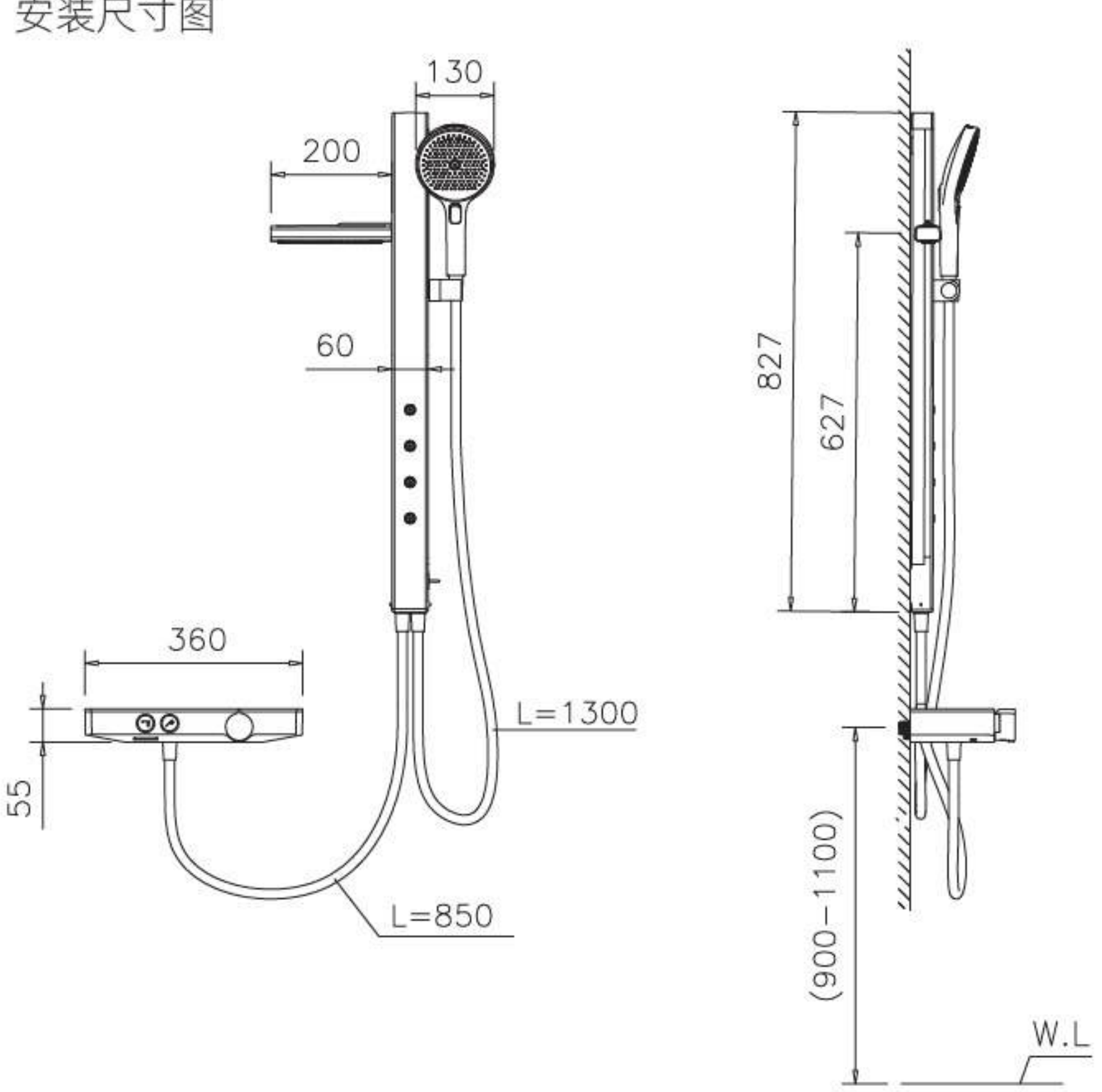
安装尺寸图
