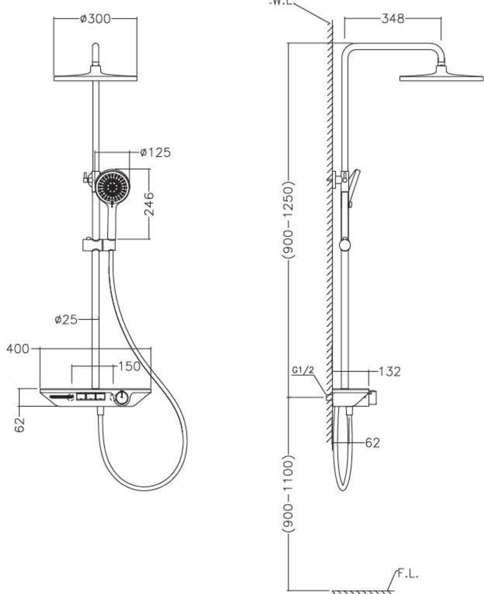
安装尺寸图
