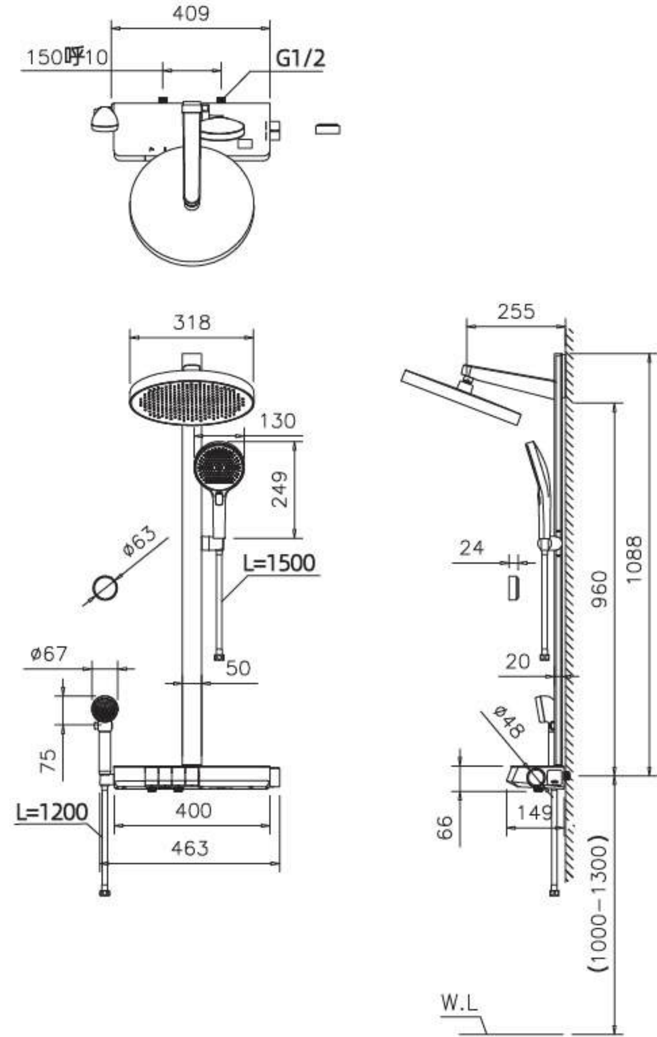
安装尺寸图
